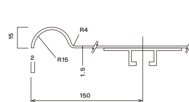
A-A' 断面
